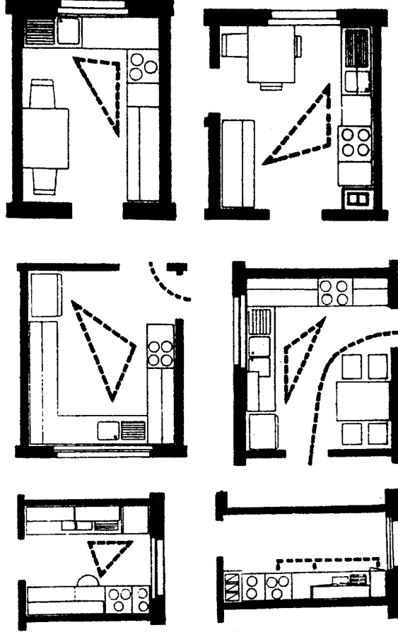
Şekil 6. Değişik mutfak tiplerinde kullanım anında oluşan dolaşım alanları (Ölçek 1/100)
